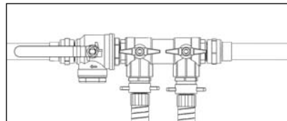
*Plnicí jednotka v normální poloze
