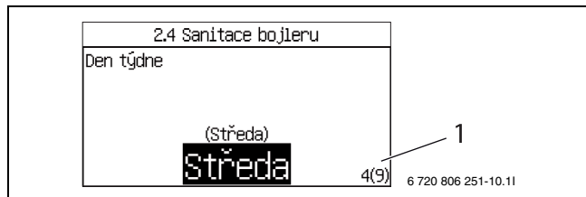
Obr. 15 Pomocná informace 3
