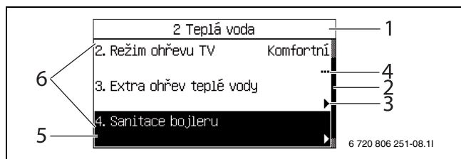
Obr. 13 Pomocná informace 1
