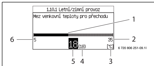
Obr. 14 Pomocná informace 2
